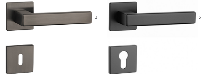
A /// rendelésre 7-10 nap TILIA F 1. PVD fényes antracit / 2. PVD matt antracit / 3. matt fekete A zamak M A=147 mm ROZ=52x52x5 mm
