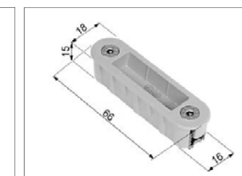
Alutop XT megfordítható zárólemez fém tokhoz
