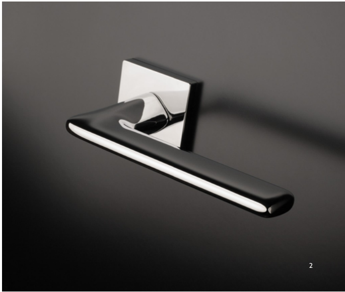
A /// rendelésre 7-10 nap LUNARIA F 1. matt króm / 2. fényes króm / 3. fényes arany / 4. szatén arany / 5. fekete A zamak M A=140 mm ROZ=52x52x7 mm
