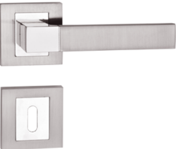
/// készleten BASIC FLORIDA F fényes króm-szatén nikkell A alumínium M A=120 mm D=52 mm | Rozetta magassága: 10 mm
