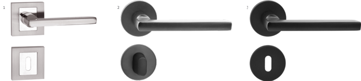
/// készleten BASIC DANIELA F fényes króm-szatén nikkell, antracit, fekete A alumínium M 1. A=117 mm D=52 mm 2-3. A=125 mm D=51 mm | Roz. mag.: 1. 10 mm 2-3. 6 mm
