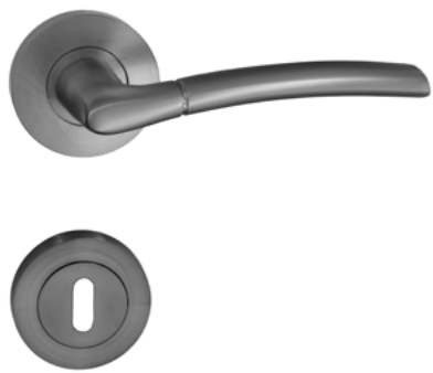
/// készleten BASIC VESTA F antracit A zamak és alumínium M A=125 mm D=54 mm | Rozetta magassága: 10 mm
